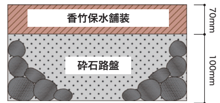
施工断面
